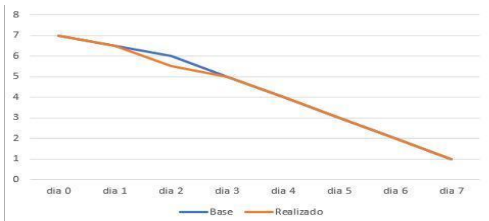
Figura 3: Burndown Sprint 1
